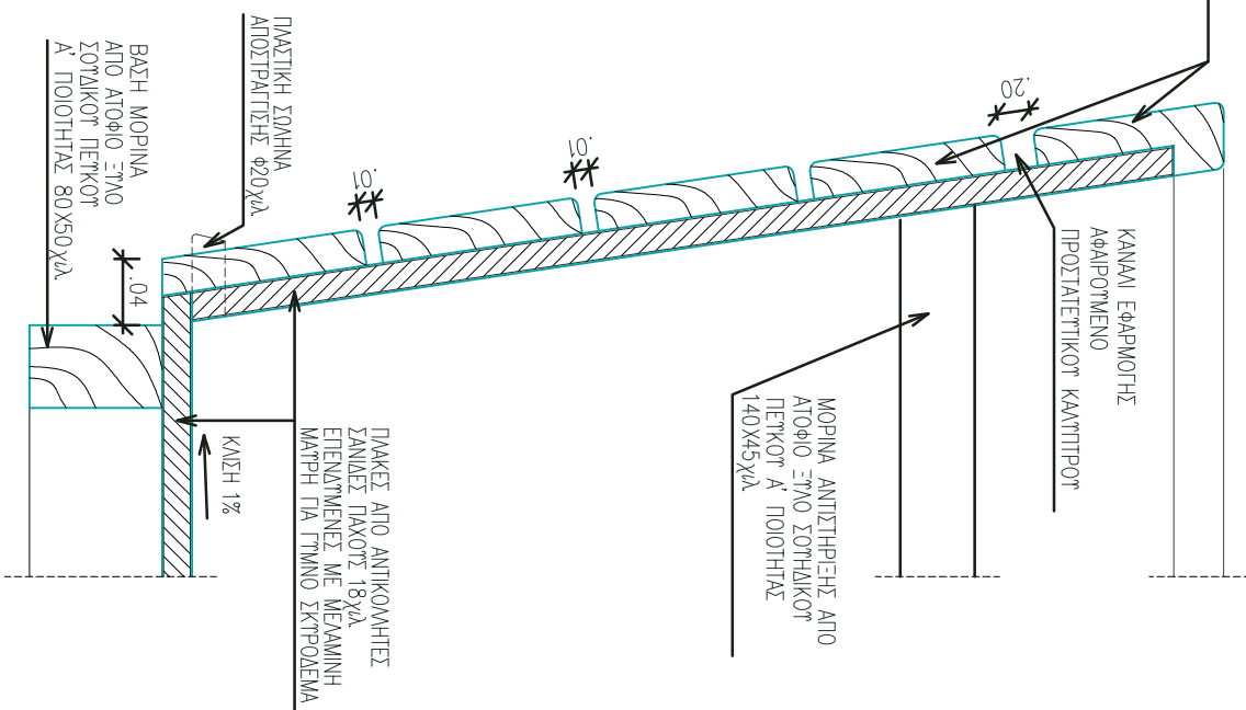
ΑΕΠΤΟΜΕΡΕΙΑ ΤΟΜΗΣ α-α ΚΑΜΑΚΑ: 1:5
