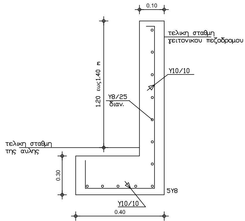
Τοίχος Αντιστηριξης ΤΑ1 κλίμακα 1: 20
