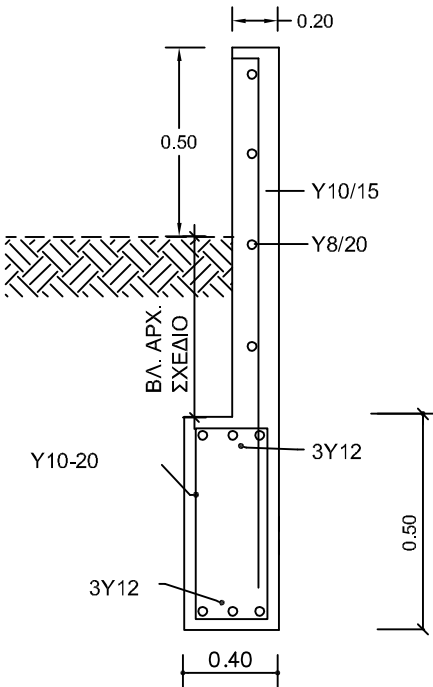
ΛΕΠΤΟΜΕΡΕΙΑ ΣΙΔΕΡΟΣΥΝΔΕΣΗΣ ΣΔ1 ΚΛ. 1:20
