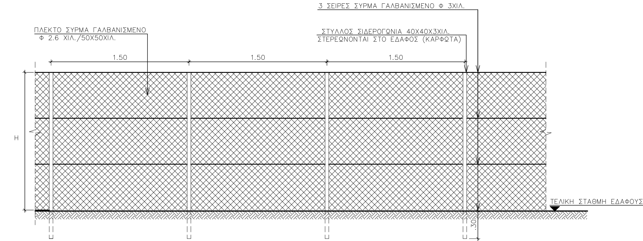
ΤΥΠΟΣ Α : ΠΡΟΧΕΙΡΗ ΠΕΡΙΦΡΑΞΗ (ΕΠΙΠΡΟΣΘΕΤΑ ΓΙΝΕΤΑΙ ΚΑΙ ΕΠΕΝΔΥΣΗ ΜΕ ΠΡΑΣΙΝΗ ΚΑΝΝΑΒΙΤΣΑ) ΚΛ. 1:25
